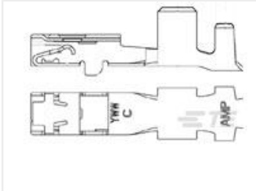
TE 产品编号1326030-7 2.8MM RECP,UNSEAL,14-16AWG,REV
