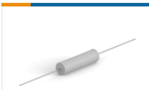
TE 产品编号8-2176414-4 7W STD M/OX 5% 56K
