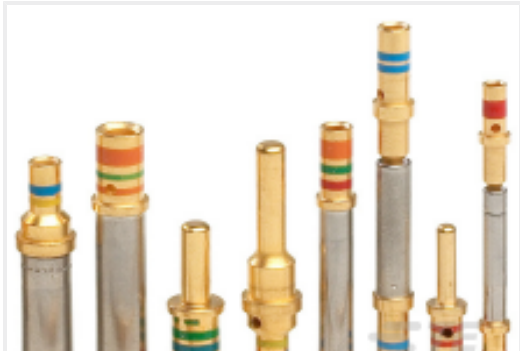
TE 产品编号ZPF000000000000570 020-0511-20
