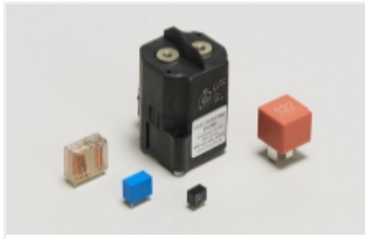
机电继电器(123)
