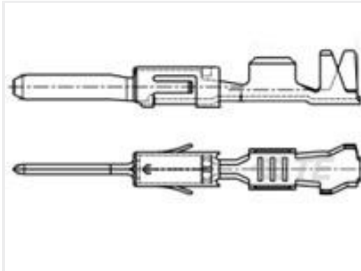
TE 产品编号963904-3 TAB A 1.6x0.6 CONTACT CS SWS Au
