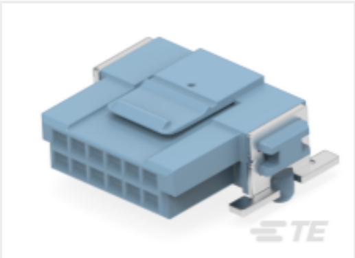
TE 产品编号254262-E SMCQ 12 F AB VV 7-03 CL * 0007 137 E002
