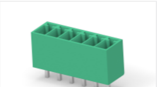
TE 产品编号 2351886-6 6POS TB HDR 180 DEG, PITCH 3.5, TL 3.4mm
