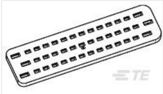
TE 产品编号963225-1 DICHTUNG F 42P GEH
