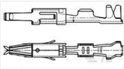
TE 产品编号963711-2 MICRO TIM RECEPTACLE CONTACT
