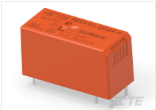
TE 产品编号8-2158000-4 RZ01-1CL-D024-R
