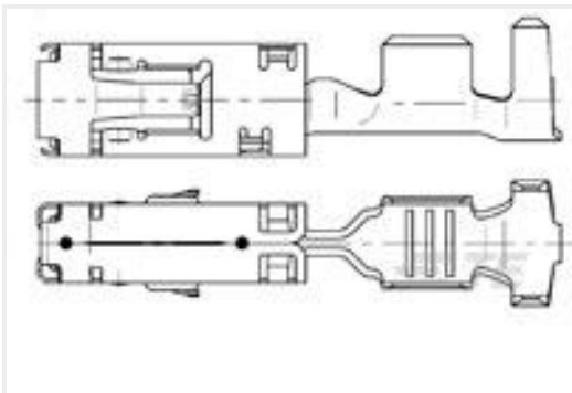
TE 产品编号967542-2 SENS FLA-KONT 2,8
