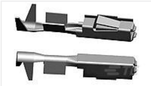
TE 产品编号5-968221-6 MQS0,63 Ag rec CB unseal. 0,5-0,75
