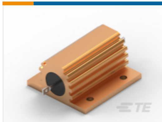
TE 产品编号6-1625971-3 功率电阻器：铝壳体，HSA
