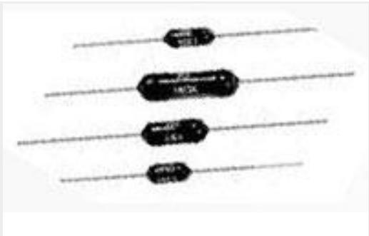
TE 产品编号8-1879663-5 H8 806R 0.1% 15PPM
