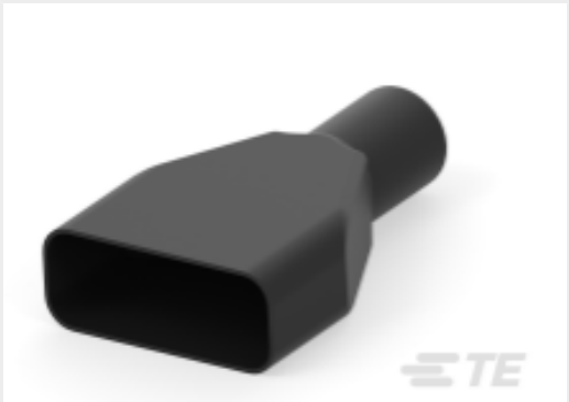
TE 产品编号DRC26-40BT BOOT, 40P, 20SZ, PLG/REC, ST, BLK
