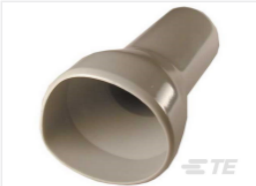
TE 产品编号HD30-24BT BOOT, 24SZ, ST, GRY
