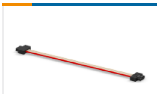
TE 产品编号839016-E IDCCS SRC 1,27 4 * SFX SFX 100 PVC
