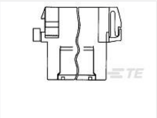
TE 产品编号929505-7 FF FA-STE-GEH2X11P
