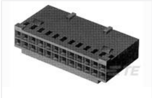
TE 产品编号87631-5 10 MODIV HSG COMP DR .100 POL
