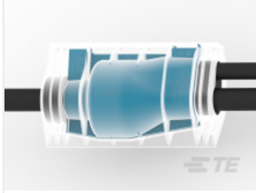
TE 产品编号 EE8510-000 MM-5-3D170-SRC4
