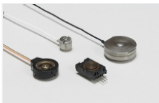
力传感器(19)
