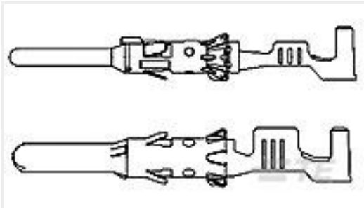
TE 产品编号929965-1 STIFTKONTAKT 2,5MMD
