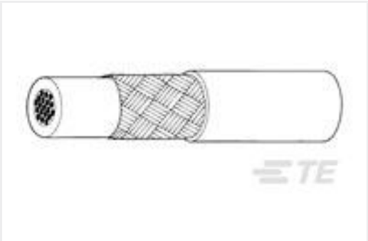
TE 产品编号172071-000 82A1111-24-9-9
