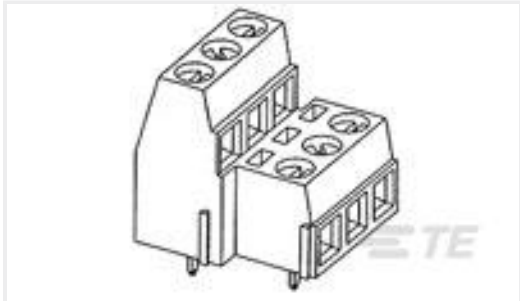
TE 产品编号CB2528-000 HVT-Z-253/353-J
