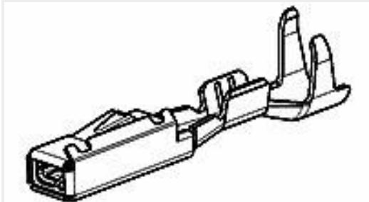
TE 产品编号1355553-1 MQS1,5 Sn rec LL unseal. 0,75-1,5
