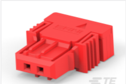
TE 产品编号364201-E SRCBUG A 2,54 2 2 CSI 165 E1 ADV TRAY J
