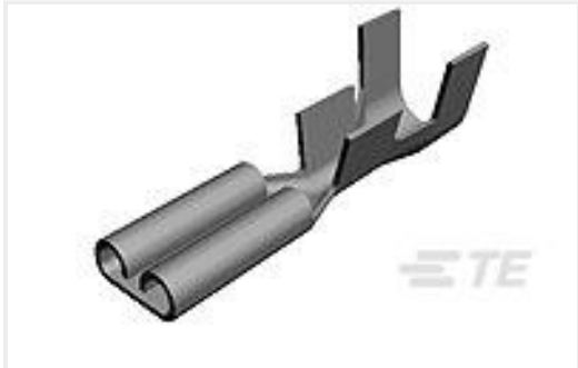
TE 产品编号63705-1 125 FASTON REC 22-18 AWG BR
