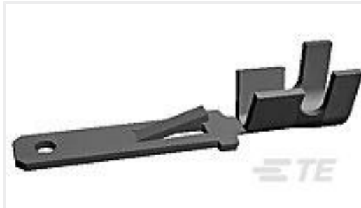
TE 产品编号170014-5 FF 110 TAB 20-16AWG BR
