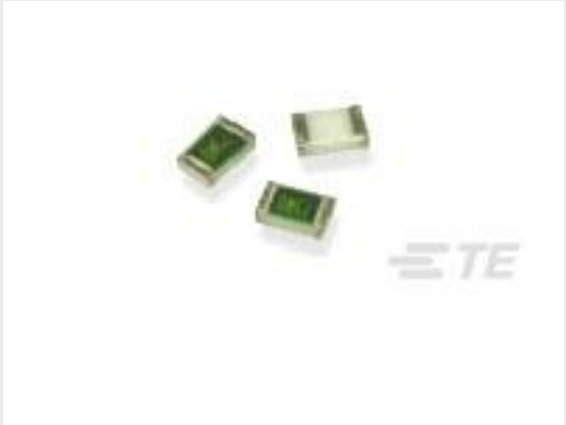
TE 产品编号2-2176094-6 RP 2A 0.25W 221K 0.1% 25PPM 1K RL
