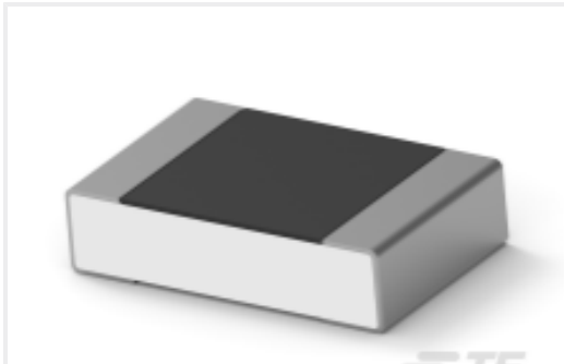
TE 产品编号1-2176376-8 RQ 0805 18K7 0.1% 10PPM 1K RL
