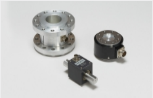
扭矩传感器(25)
