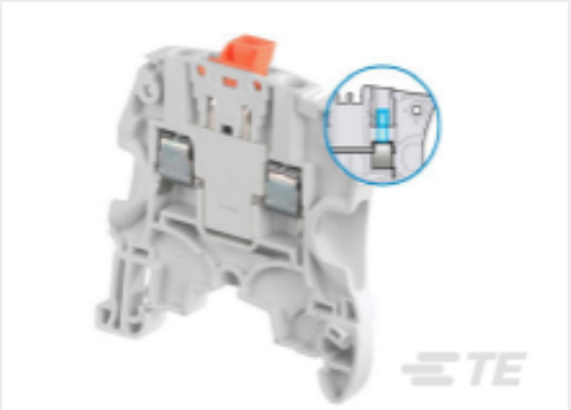
TE 产品编号1SNK505312R0000 ZS4-S-T2.3
