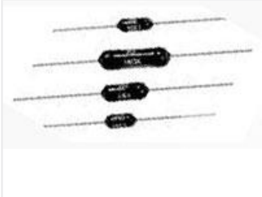
TE 产品编号9-1879663-4 H8 1K0 0.1% 15PPM
