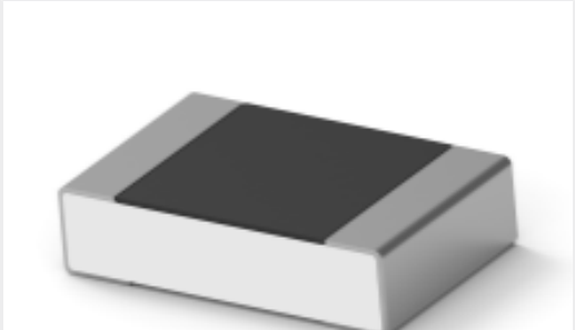
TE 产品编号9-2176373-5 RQ 0805 95R3 0.1% 10PPM 1K RL
