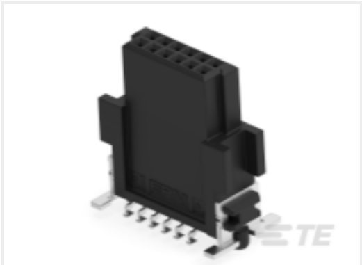
TE 产品编号494543-E SMCB 12 F AB VW 7-23 CL * 9999 137 E002
