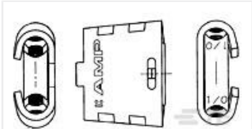
TE 产品编号83592-2 MINIWEDGE,SYM,1/0-#2,CORE
