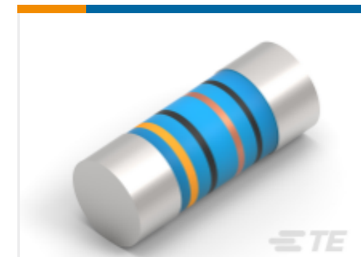
TE 产品编号9-2176314-2 MELF SMA-A 560K 1% 50PPM 0102 0.3 W
