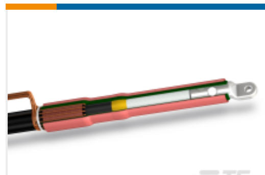
TE 产品编号A00805-064 POLT-12D/1XI
