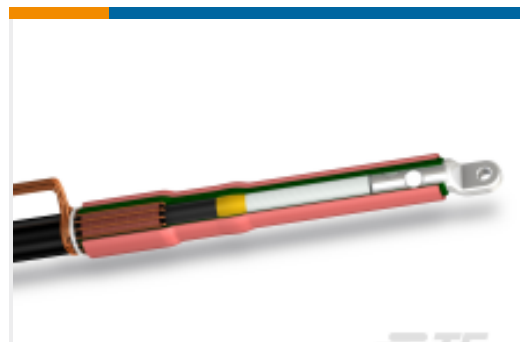
TE 产品编号914019-064 POLT-12D/1XI-L12A
