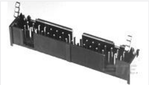
TE 产品编号1761608-3 IDC LOW PRO HDR 10P VERT SHT L
