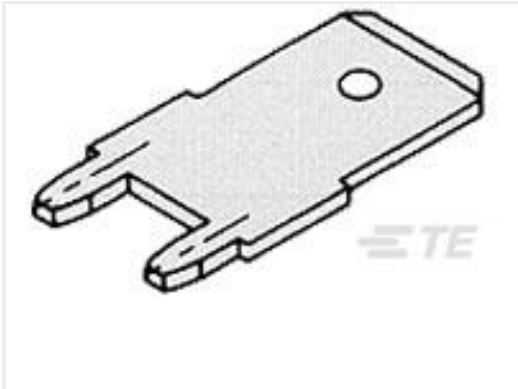
TE 产品编号62409-1 250 FASTON TAB TPBR
