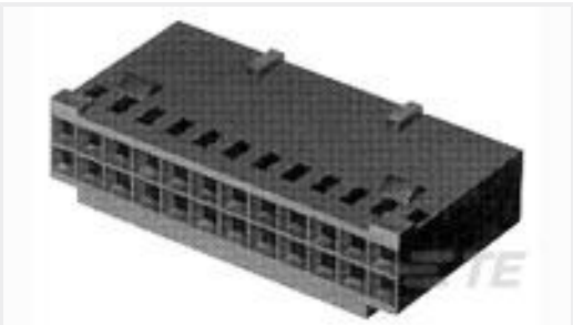
TE 产品编号3-87631-1 36 MODIV HSG COMP DR .100 POL
