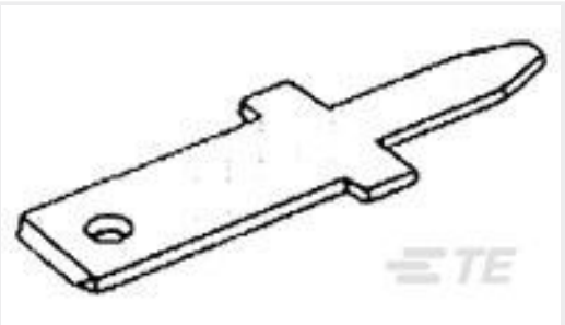
TE 产品编号63756-1 110 FASTON TAB TPBR
