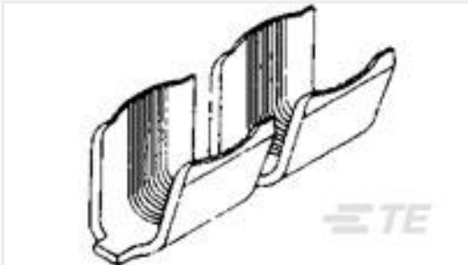
TE 产品编号42778-2 SPLICE AMPLIVAR 600-3000 CMA
