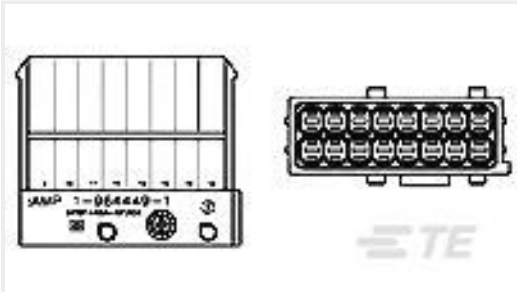
TE 产品编号1-964449-1 FLACHSTE-GEH2,8 16P
