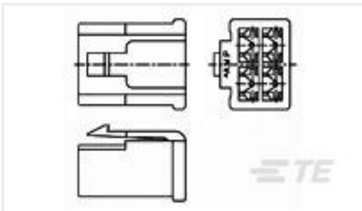
TE 产品编号174202-1 250 FASTON HSG.,REC.,4 POS, NATURAL
