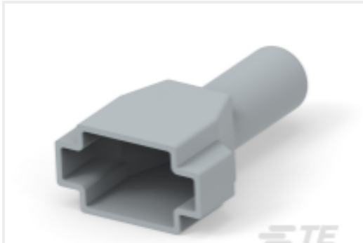
TE 产品编号DT8S-BT BOOT, 8P, PLG, ST, GRY
