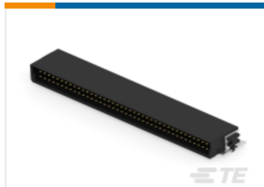
TE 产品编号154767-E SMCB 80 M AB VV 7-03 CL * 0007 137 E004
