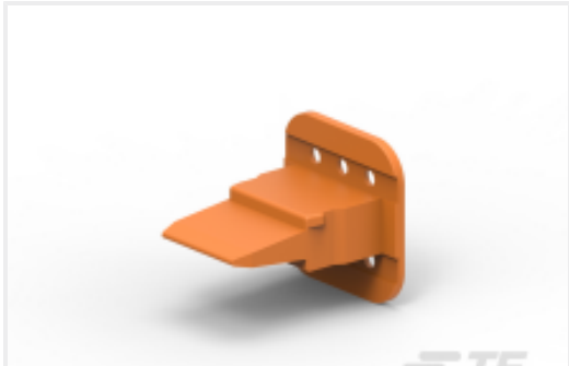
TE 产品编号W6S WEDGE LOCK, 6P, PLG, ORG, STD, DT
