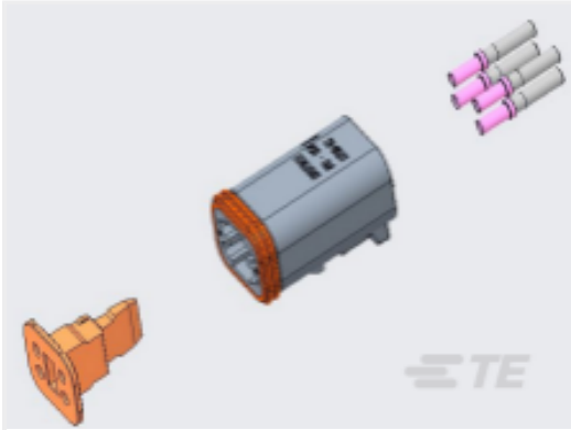
TE 产品编号DT06-4S-COMPLETE DT06-4S CON AND WEG
