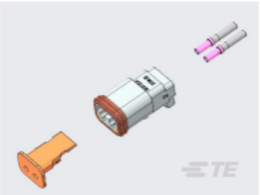
TE 产品编号DT06-2S-COMPLETE DT06-2S CON AND WEG
