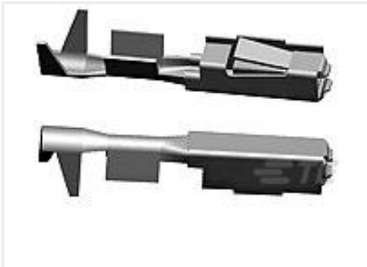
TE 产品编号5-965906-5 MQS0,63 Au rec LL EDS 0,5-0,75
