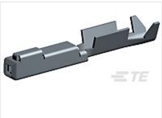
TE 产品编号2040168-2 0.64 RCPT SEALED AU STRIP(L SIZE)
