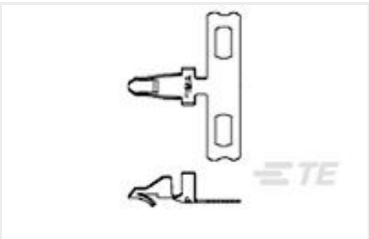
TE 产品编号3-350566-1 MINI AMP-IN 22-18 PTLP/PHBZ
